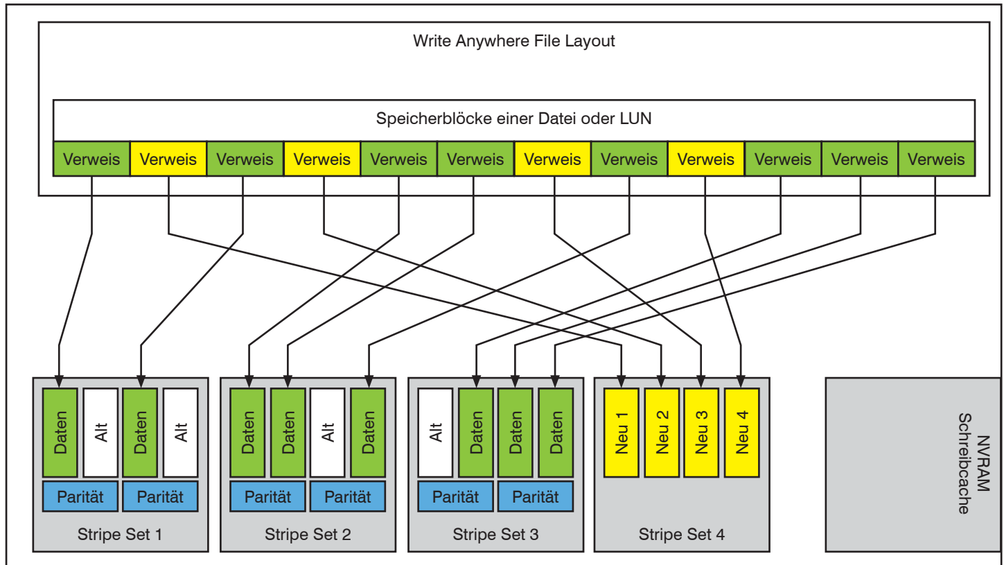
Abbildung 9: Die im Schreibcache gepufferten Daten werden in noch ungenutzte Stripe Sets geschrieben und dort um die notwendige doppelte Paritätsinformation ergänzt. Aus dem WAFL werden die Verweise von den alten auf die neuen Blöcke verlegt. Dadurch muss die Paritätsinformation in den alten Stripe Sets nicht angepasst werden. Die alten Datenblöcke bleiben erhalten und bilden einen Snapshot des ursprünglichen Datenstandes.
