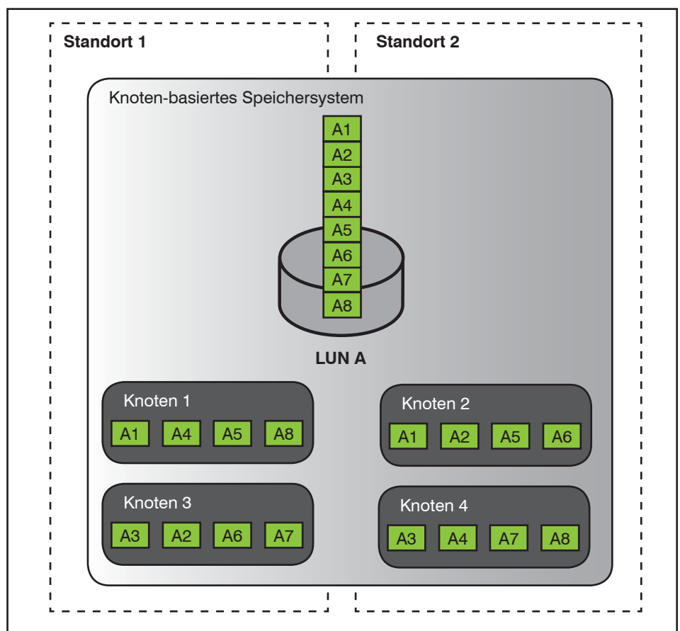
Abbildung 18: Durch eine geeignete Verteilung der einzelnen Knoten des Netzwerk-RAID10-Verfahrens entsteht eine redundante Topologie, die den Ausfall eines kompletten Standorts kompensiert und dabei einen transparenten Failover ermöglicht.
